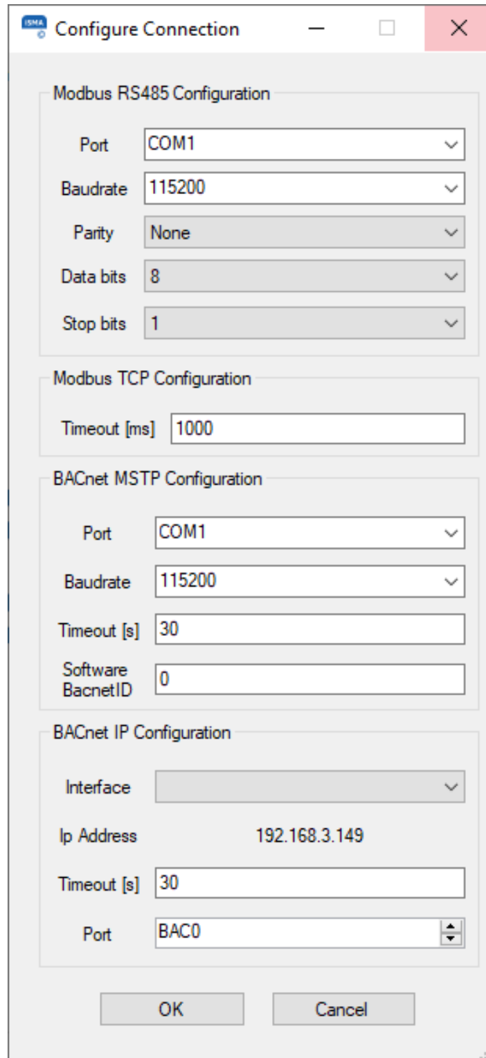
Figure 27. BACnet MS/TP configuration parameters
