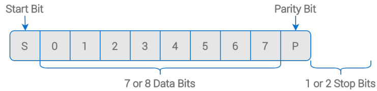
Figure 13. Modbus message frame
